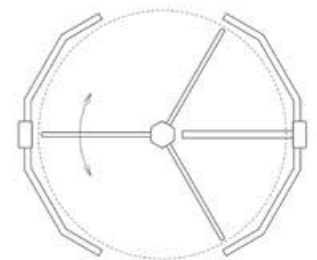
Anti-Passback-Stellung der Drehsäule mit 2. Sperrgitter
