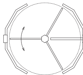
Anti-Passback-Stellung der Drehsäule mit 2. Sperrgitter
